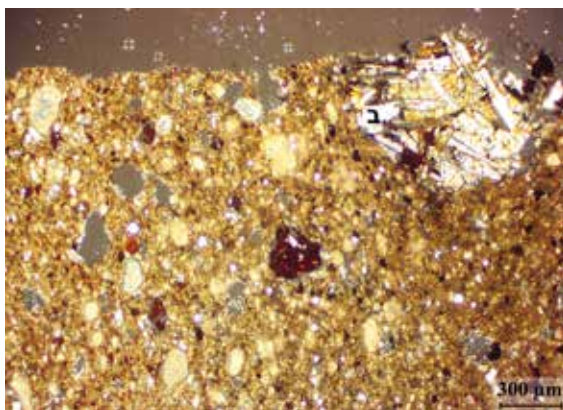
איור 6: קנקן מסוסיתא מייצור מקומי מחומר גירי עם קצת מינרלי בזלת (ב) (צילום מיקרוסקופי באור מקוטב מוצלב, מ' אזבנד).
