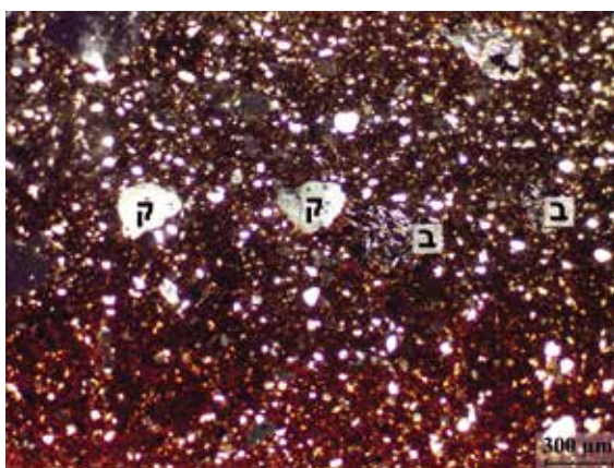
איור 7: כלי בישול מסוסיתא מייצור מקומי מחומר בזלתי עם שברי בזלת (ב), קוורץ בגודל סילט ומעט בגודל חול (ק) (צילום מיקרוסקופי באור מקוטב מוצלב, מ' אזבנד).
